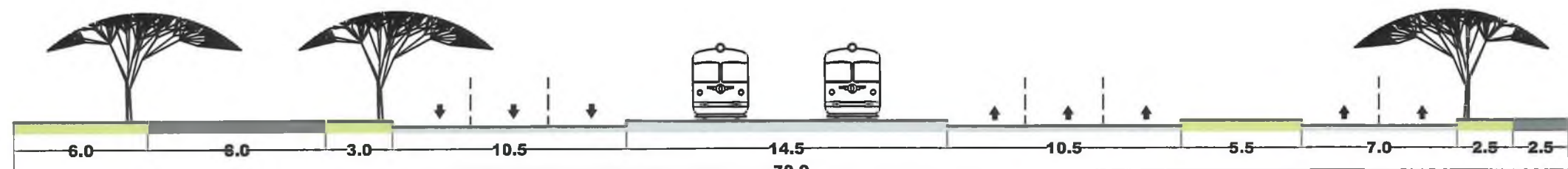
Profil Bulevardul Theodor Pallady Scara 1:250
